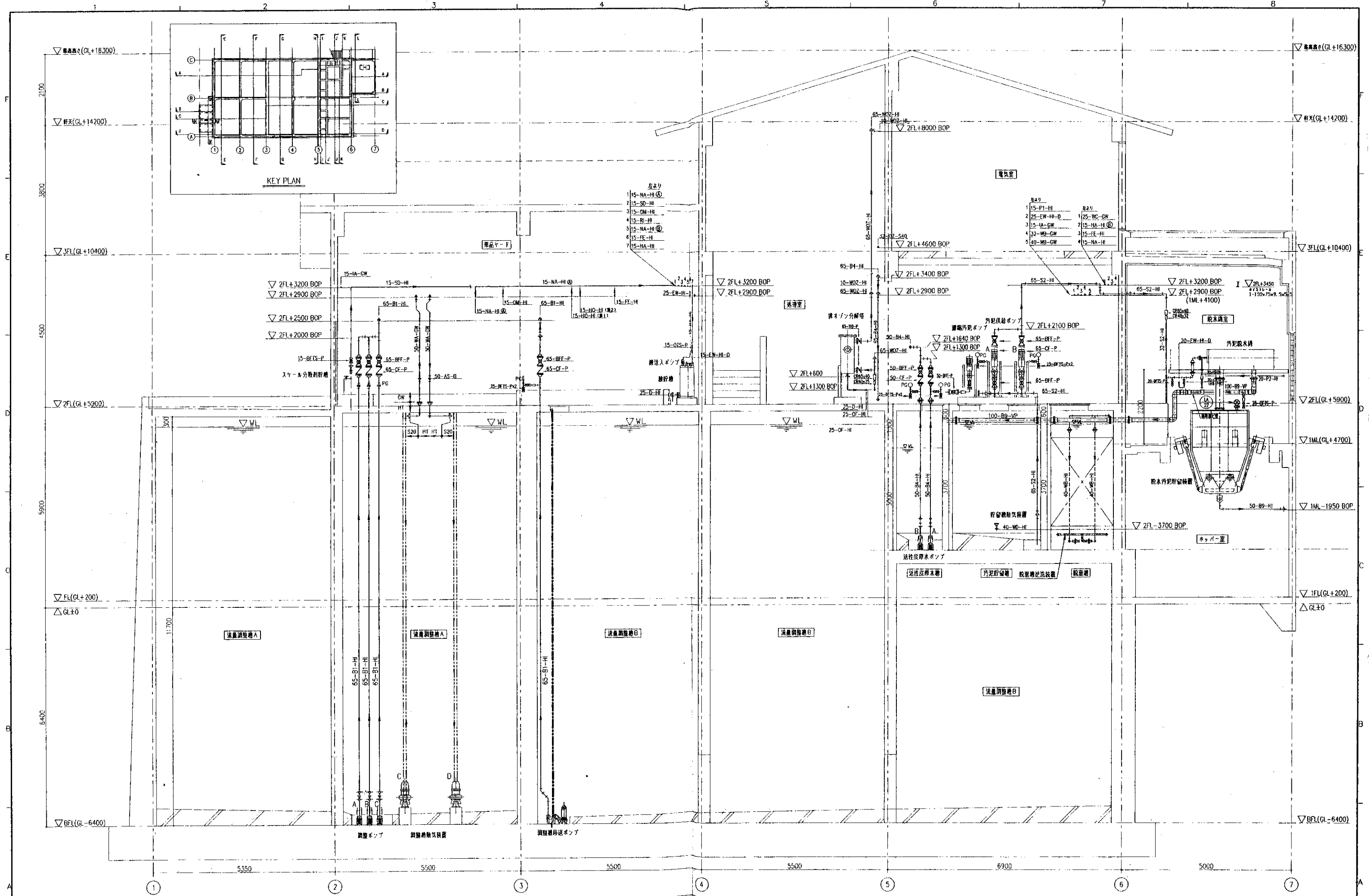
B-B断面図 1/50
